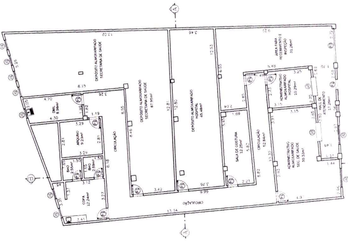
PLANTA BAIXA MODIFICADA ESCALA 1/1000
