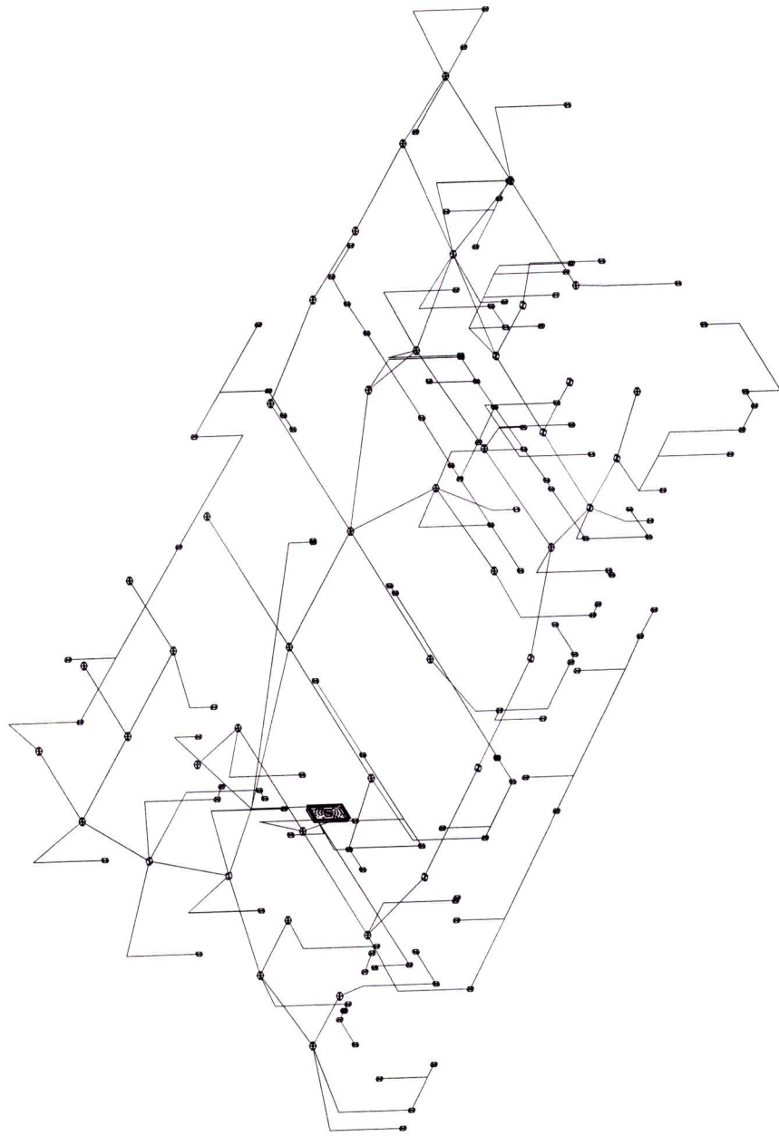
ESQUEMA ISOMETRICO DE RAÇÃO ESCALA 1 / 125
